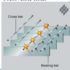
Pressveiste rister
